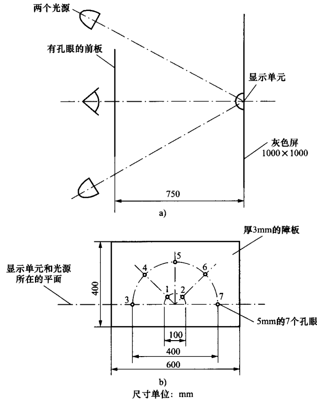
a) 俯视图; b) 前板的正视图 图3 目测显示的清晰可见度的试验布置
