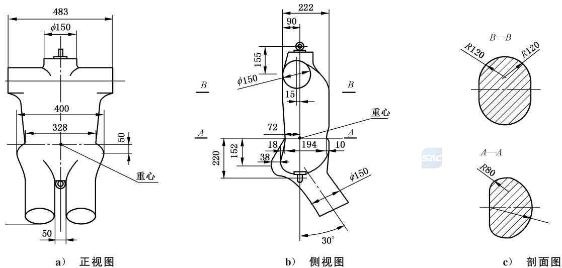
图 1 模拟人外形及主要尺寸
